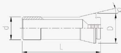
走心式筒夾
